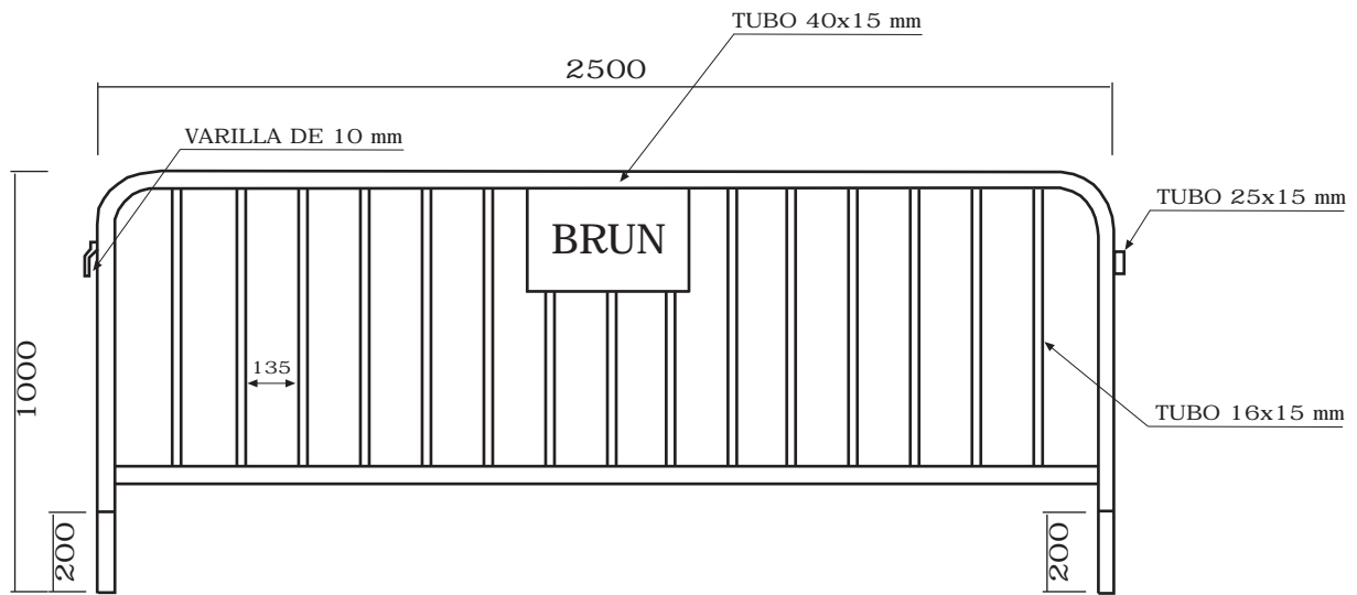
ALZADO
