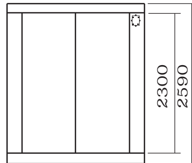
ALZADO LAT. DERECHO
