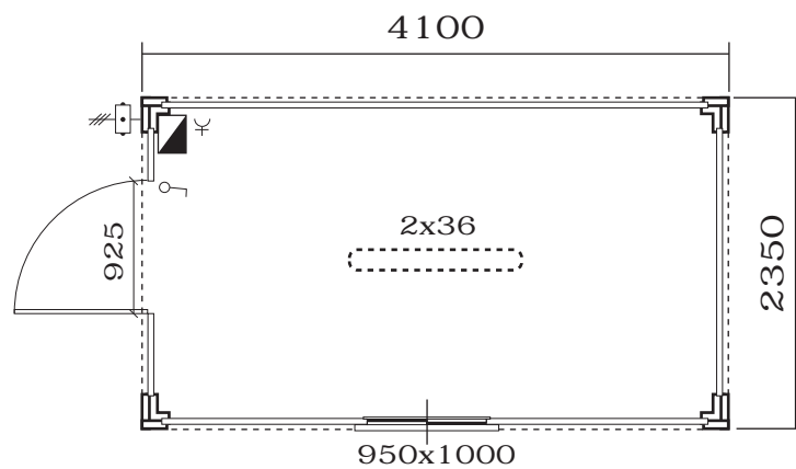
PLANTA
